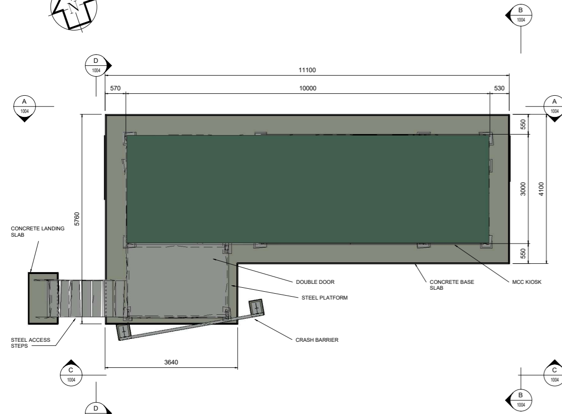
MCC KIOSK PLAN 1 : 50
