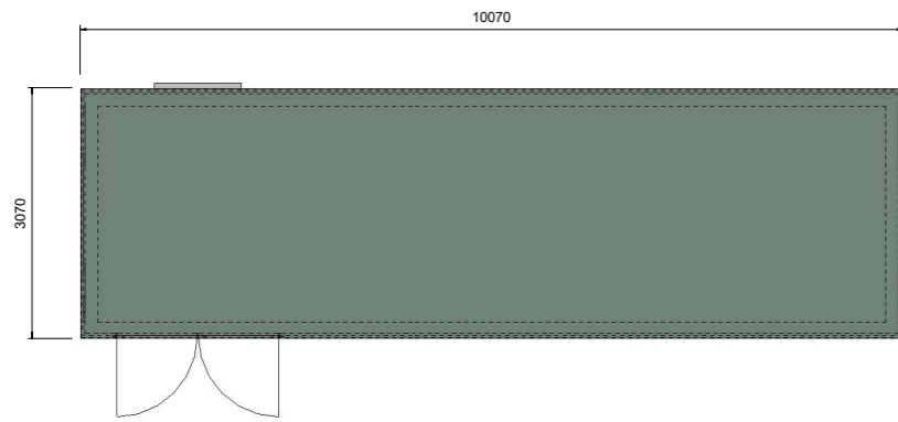
MCC KIOSK ROOF PLAN 1 : 50
