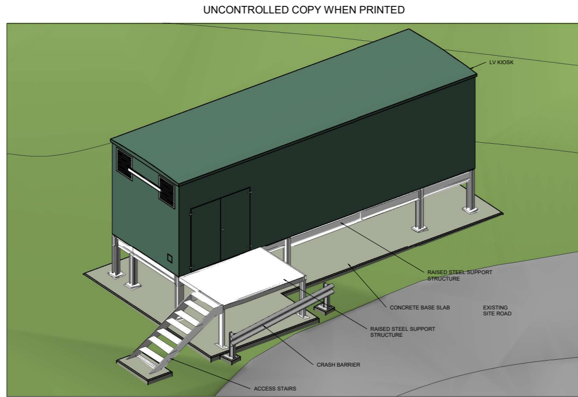
3D VISUALISATION MCC KIOSK
