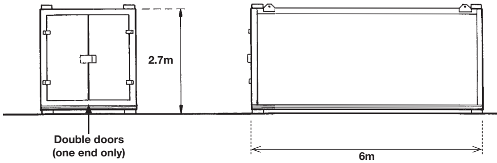
END ELEVATION
